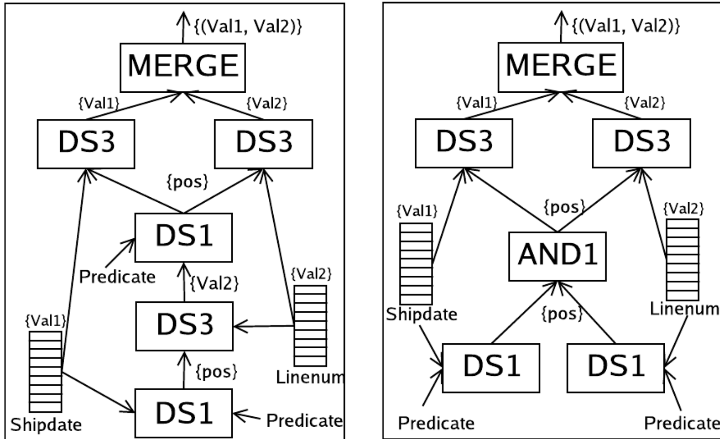
Abbildung: pipelined (links), parallel (rechts)
